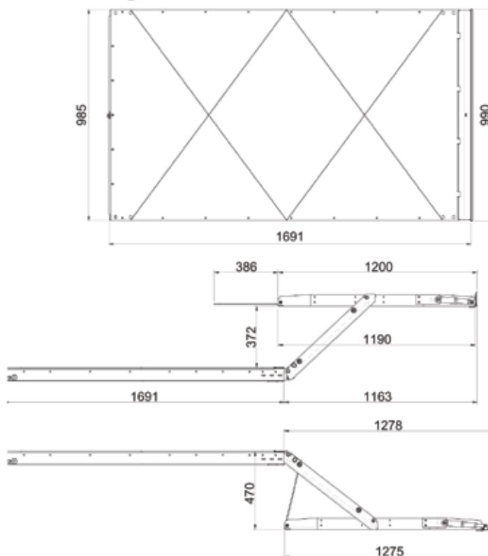
DIMENSIONS EP 300
